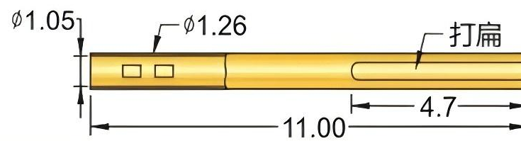
R1040 焊接片
