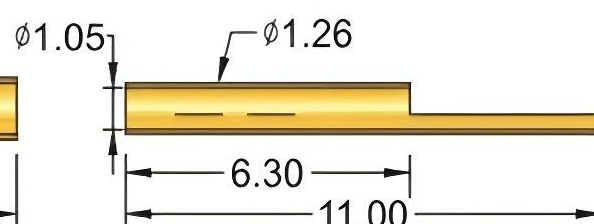
R1040 焊接片(可套用)
